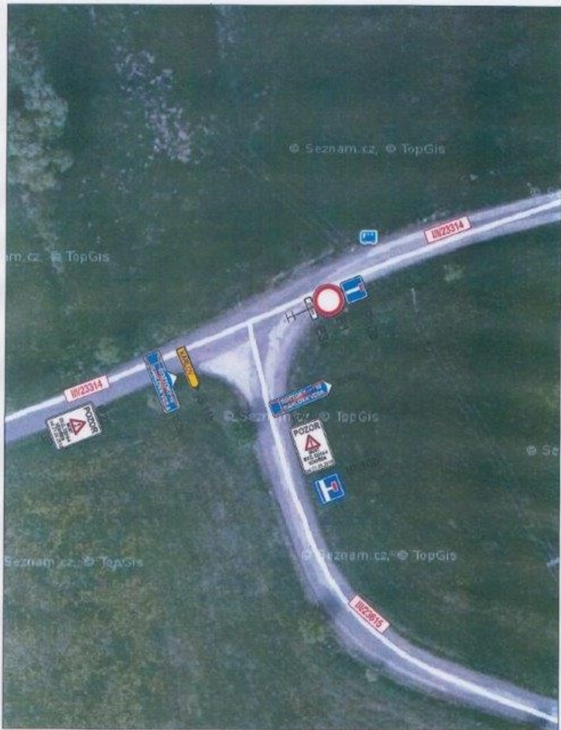
D3 - KŘIŽOVATKA III/23314 x III/23615
